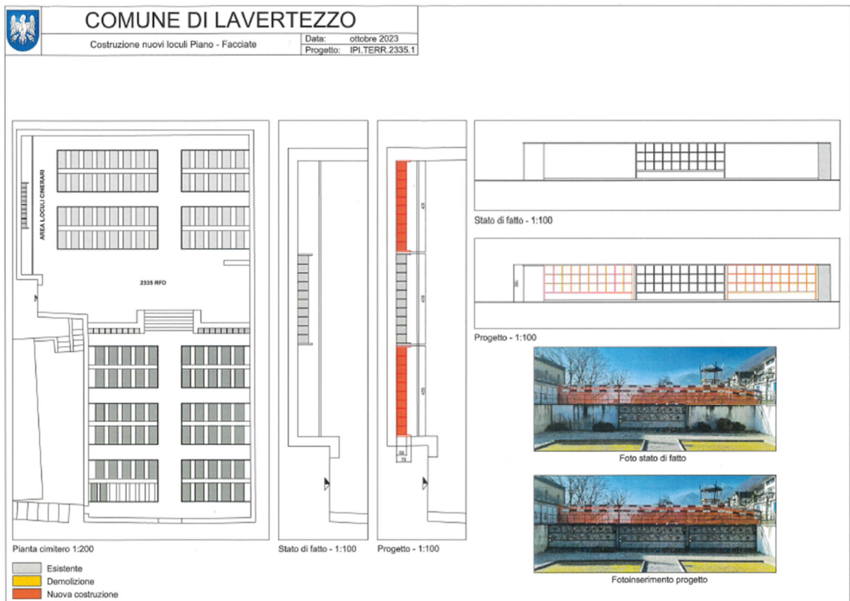
Planimetria con indicazione ampliamento in rosso Progetto nuovi loculi – UTC ottobre 2023
